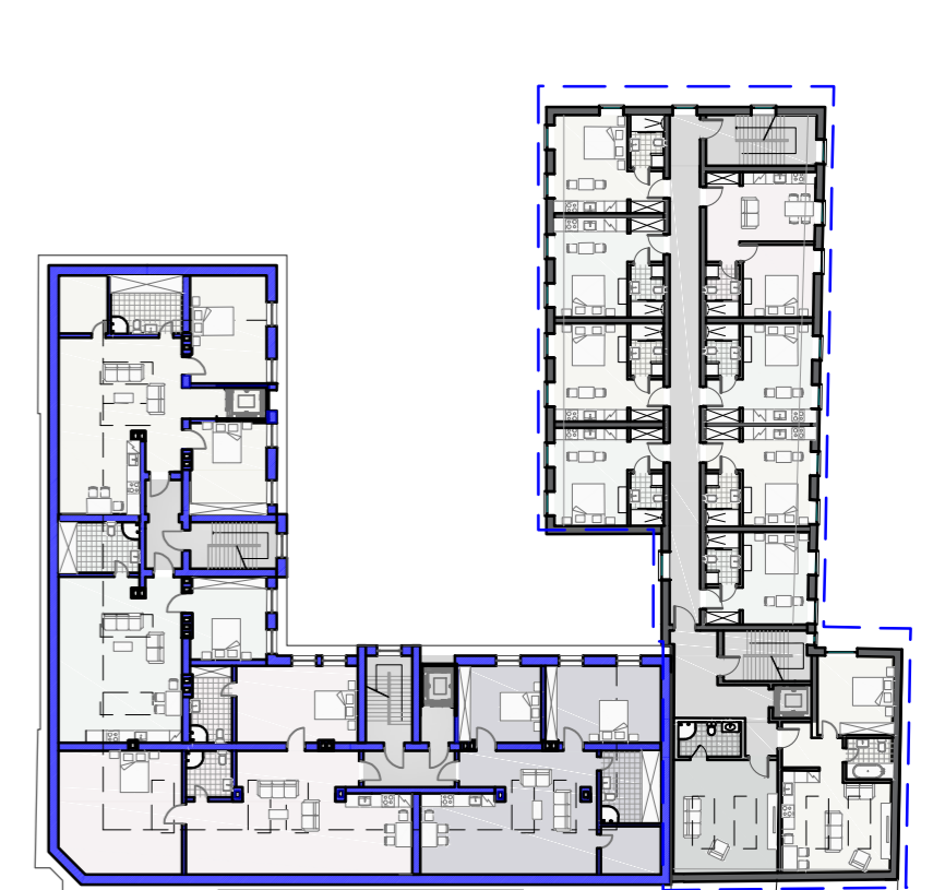
2. KĀRTA - Viesnīcas jaunbūve 5.stāvs
