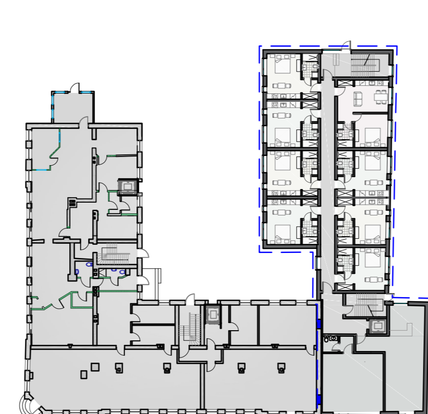
2. KĀRTA - Viesnīcas jaunbūve 1.stāvs
